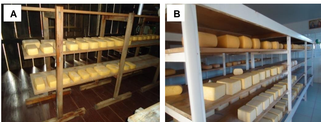
Figuras 31 – Tábuas de cura em casa de queijo de madeira (A) e casa de queijo de alvenaria (B)
